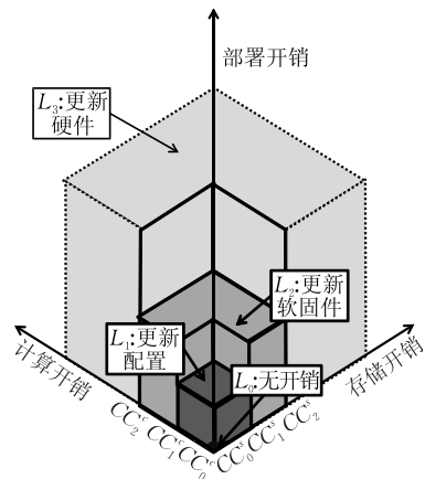
图 2 部署开销阶梯函数示意
