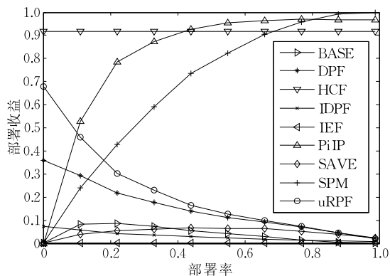
图 3 方法针对于 d-DoS 的部署收益
