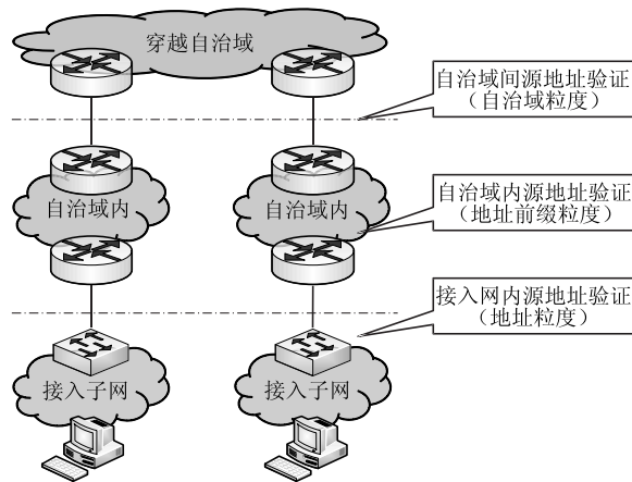
图 1 源地址验证体系结构的各个层次
