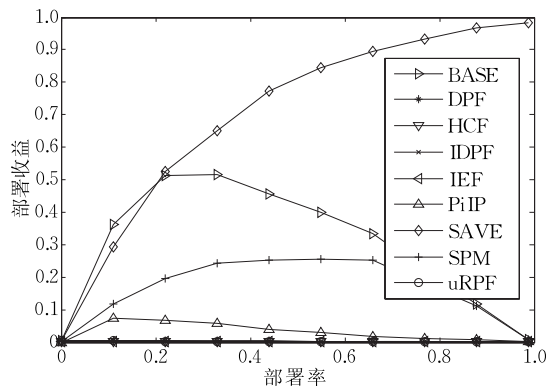
图 4 方法针对于 s-DoS 的部署收益
